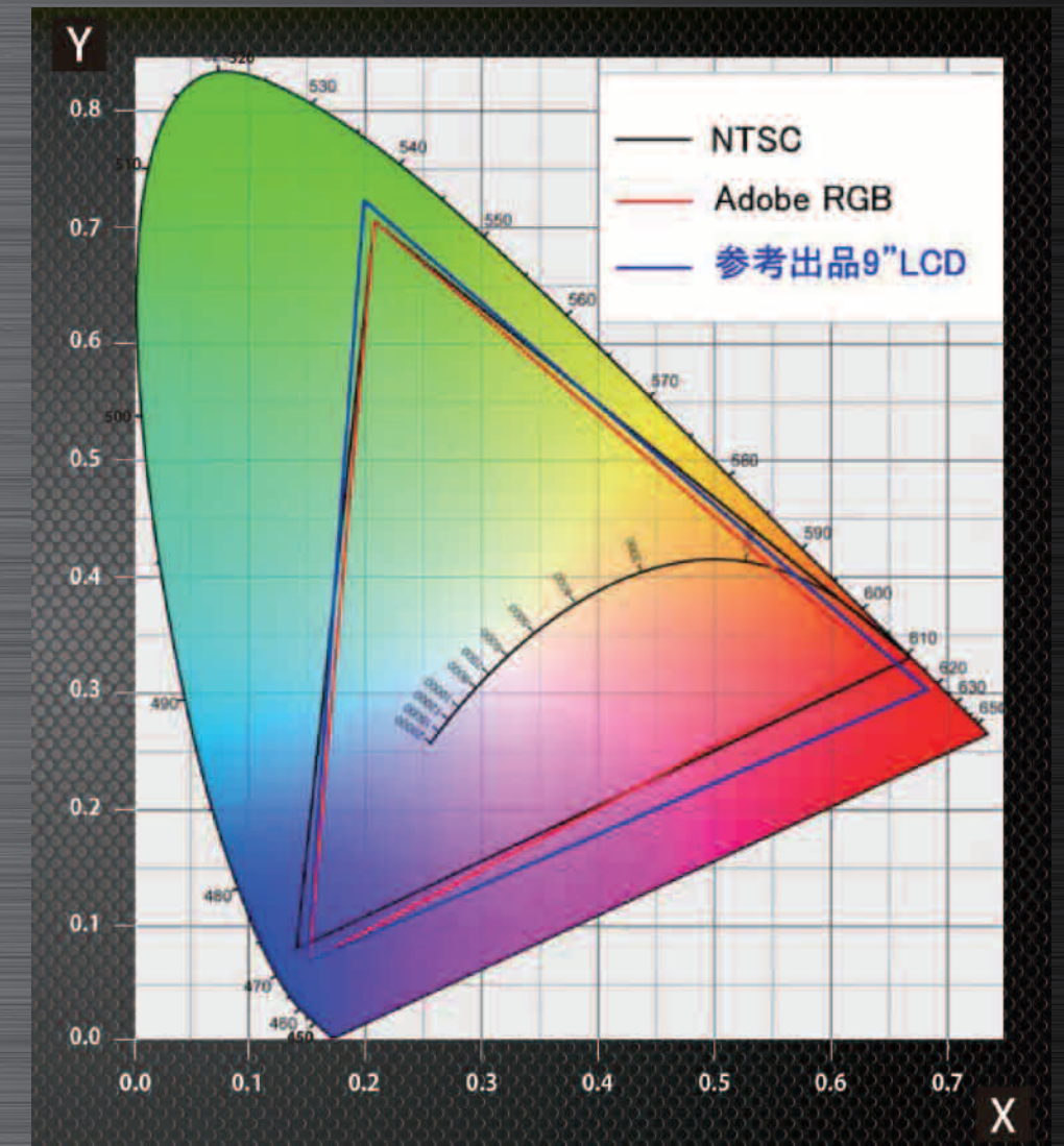
CIE1931 色度図
